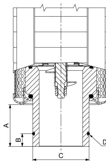
Fig. 75 Inlet pipe
